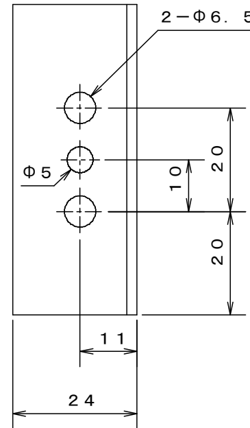
右側面 リレー仕様
