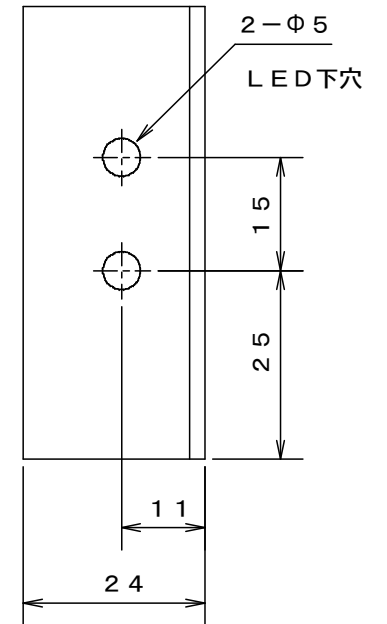
右側面 赤外線LED仕様
